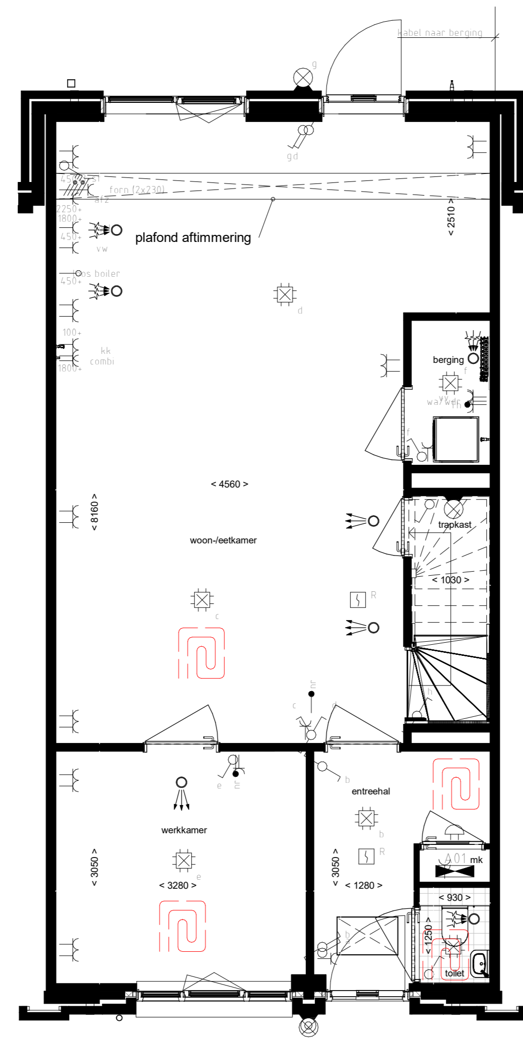
Begane grond - indeling variant B
