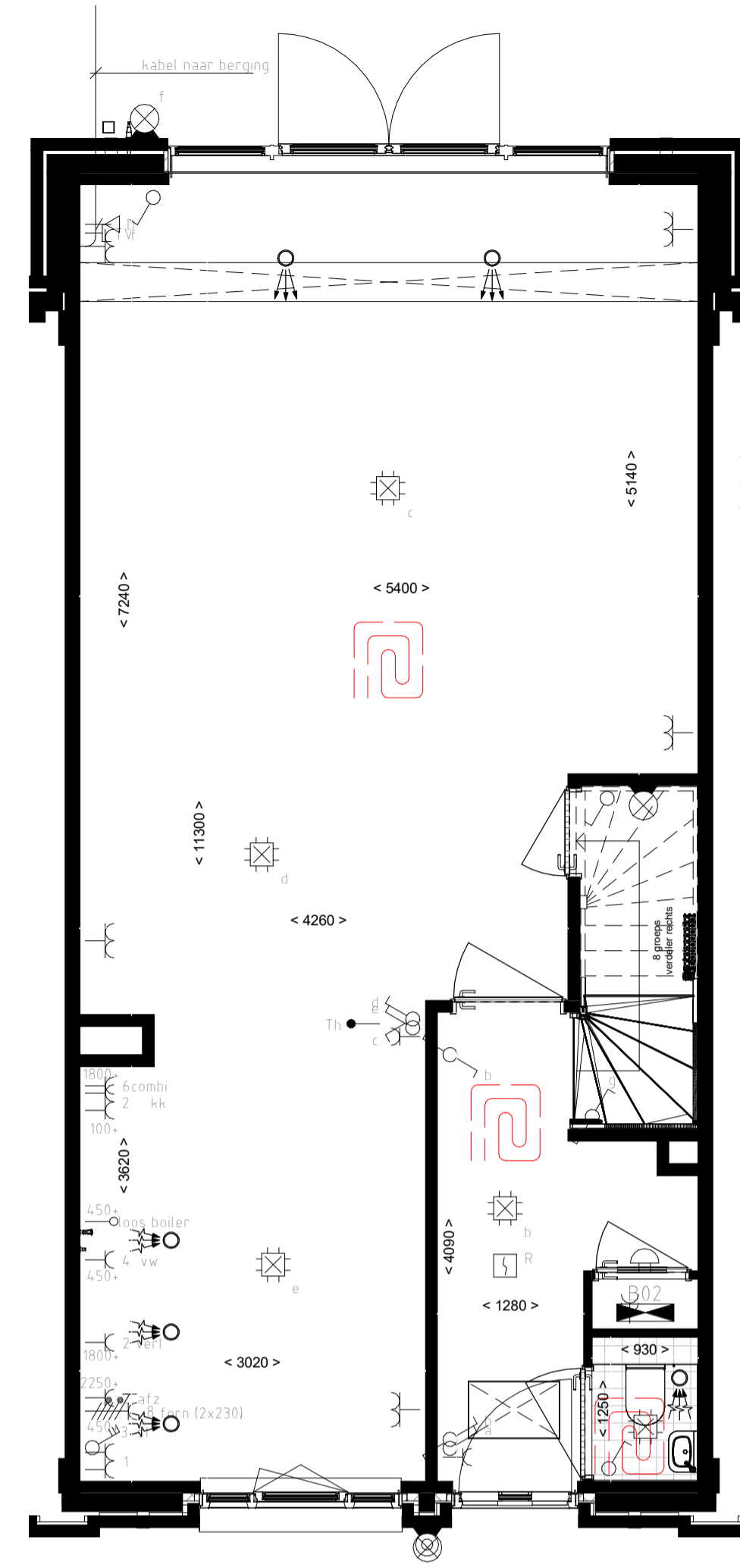
Begane grond - uitbouw 1,2m
