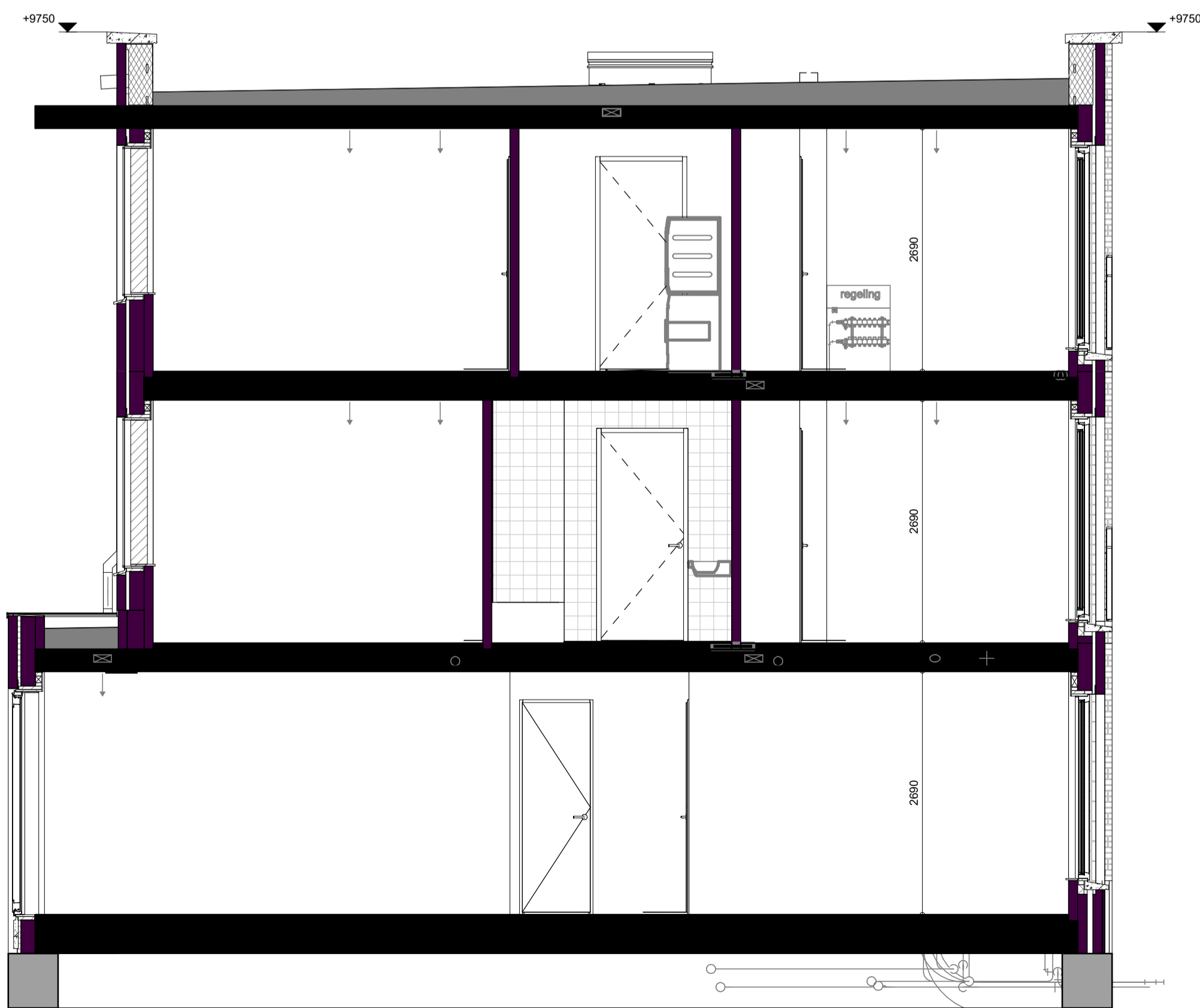
Doorsnede - uitbouw 1,2m
