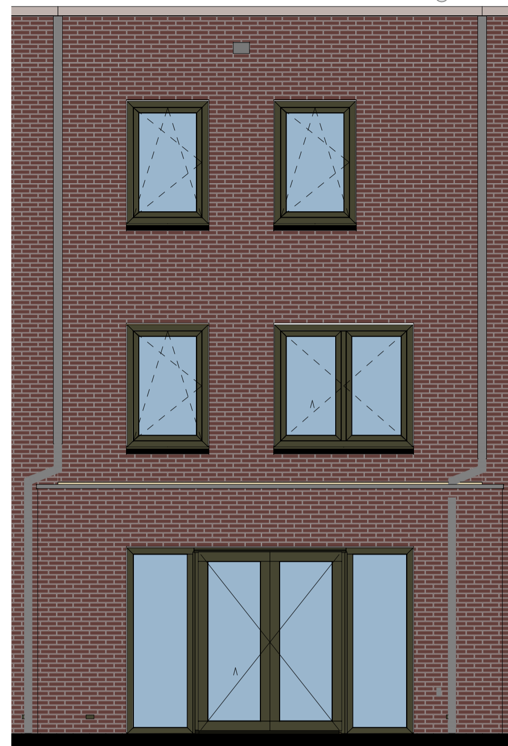
Achtergevel met uitbouw
