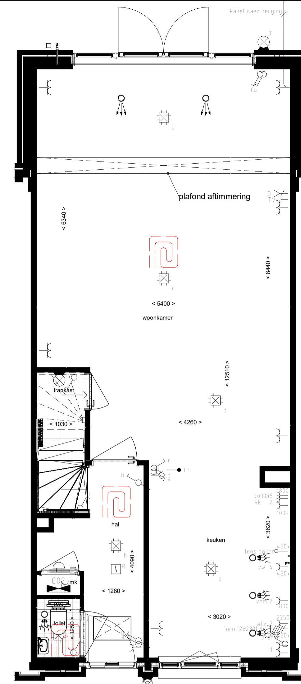
Begane grond - uitbouw 2,4m
