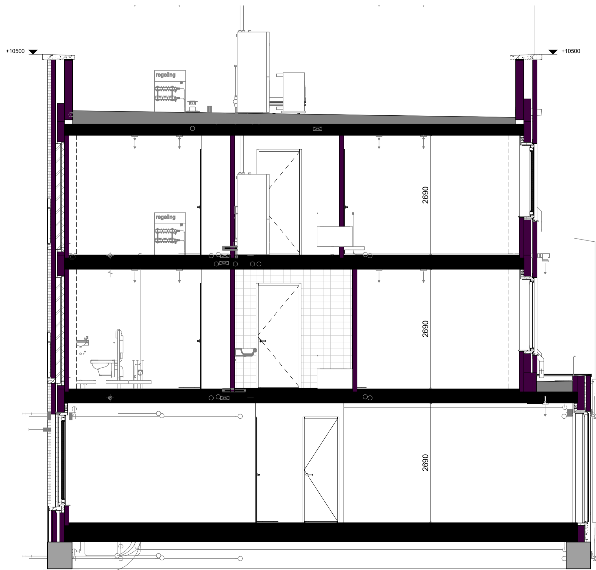
Doorsnede - uitbouw 1,2m
