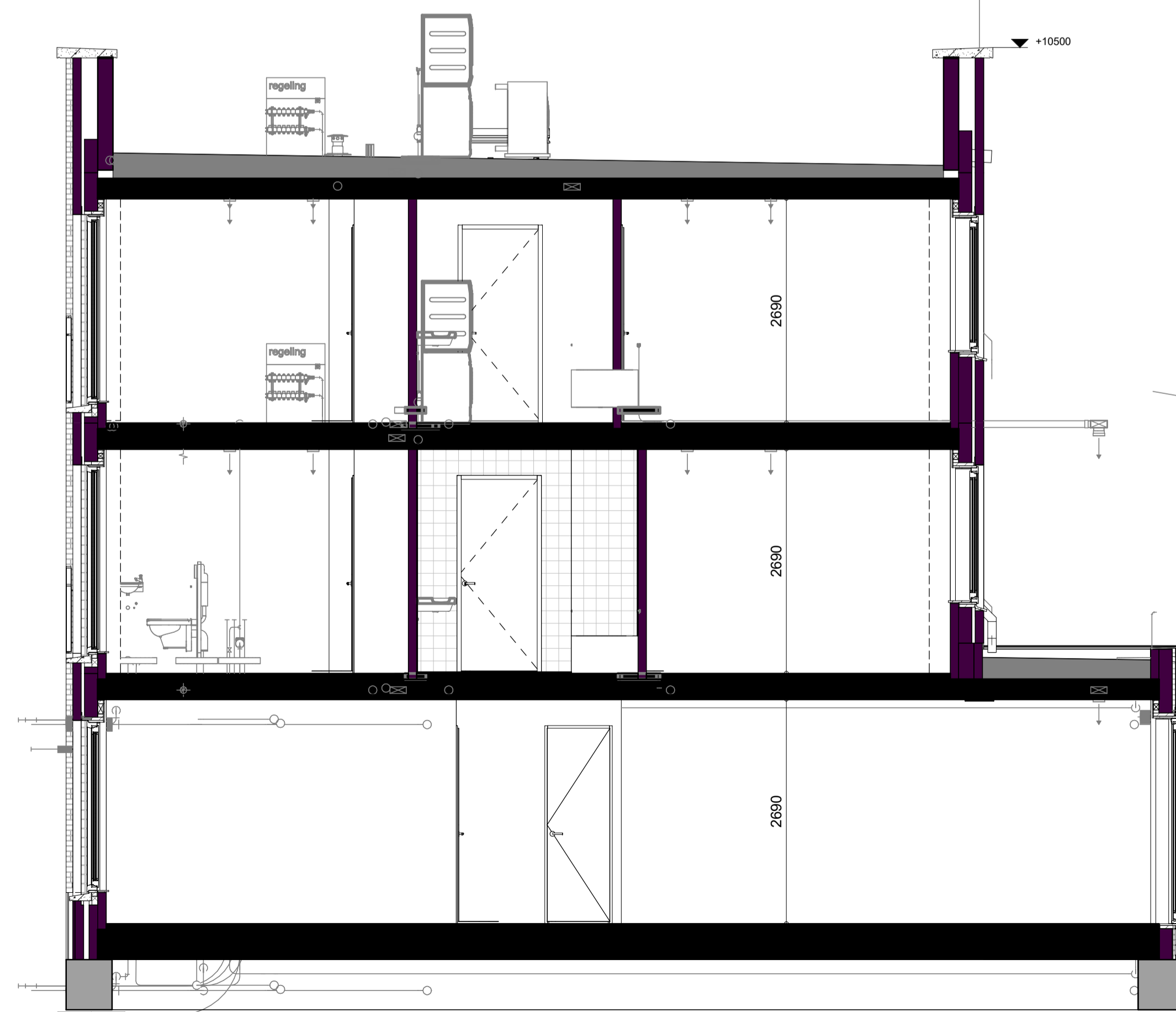
Doorsnede - uitbouw 2,4m
