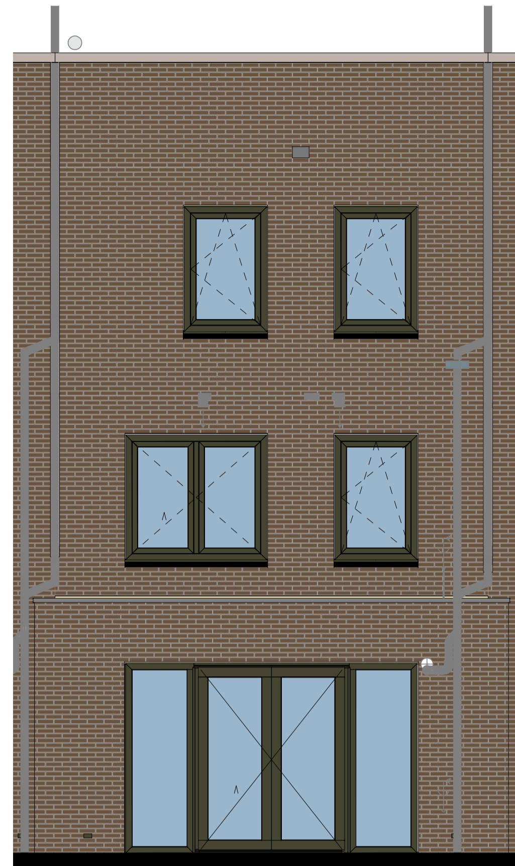
Achtergevel met uitbouw
