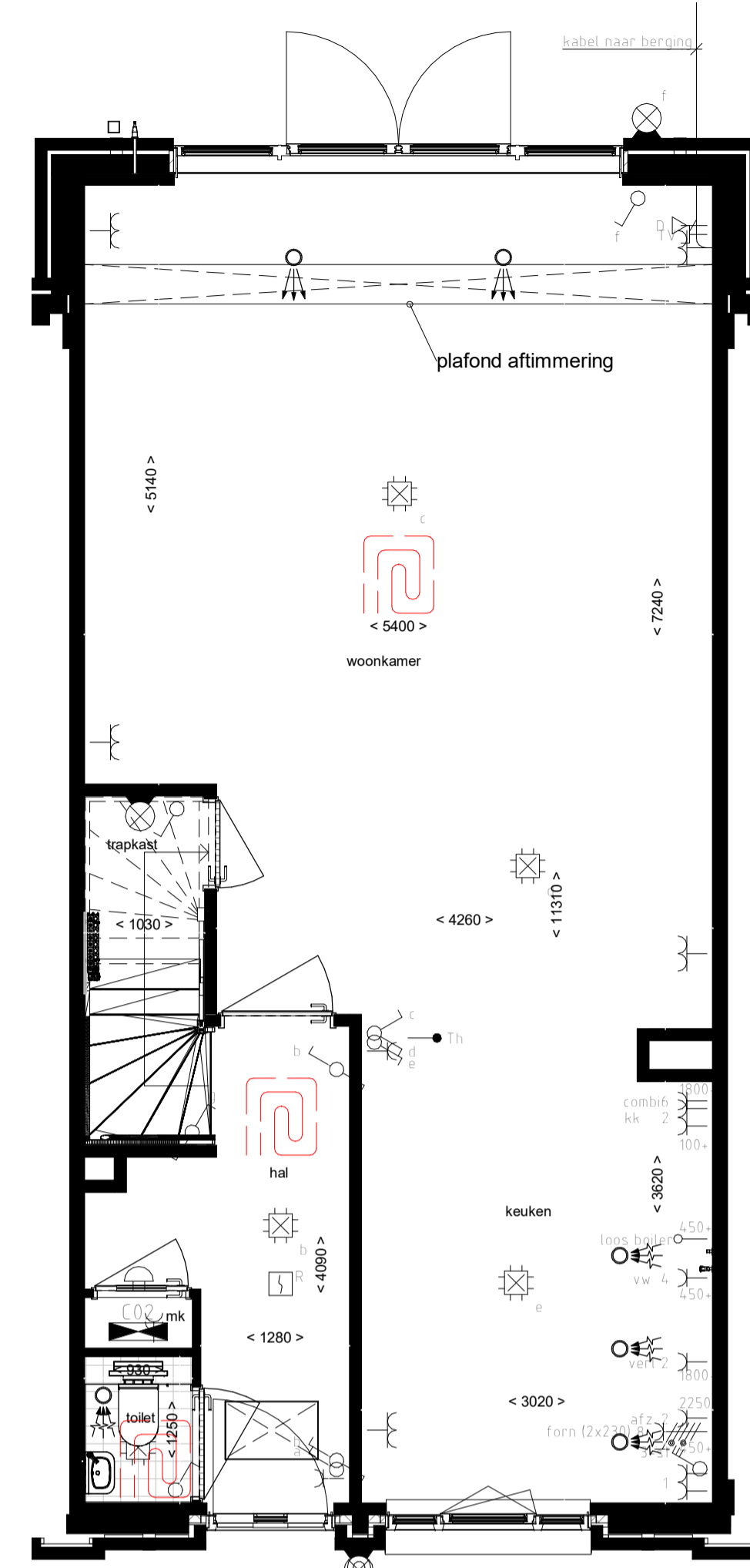
Begane grond - uitbouw 1,2m
